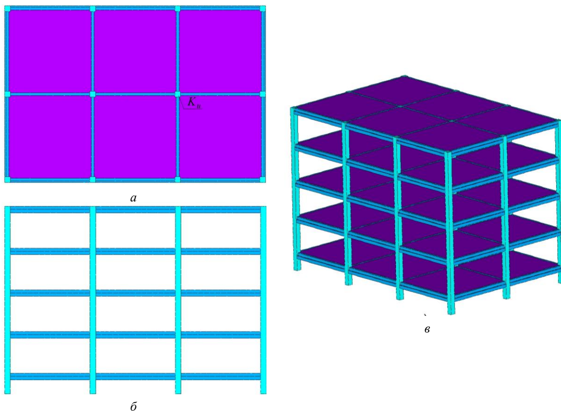
Рис. 1. Модель сборно-моноконтрукции: а – вид сверху; б – вид сбоку; в – пространственный вид; K_u – колонна, моделирующая вертикальное смещение
