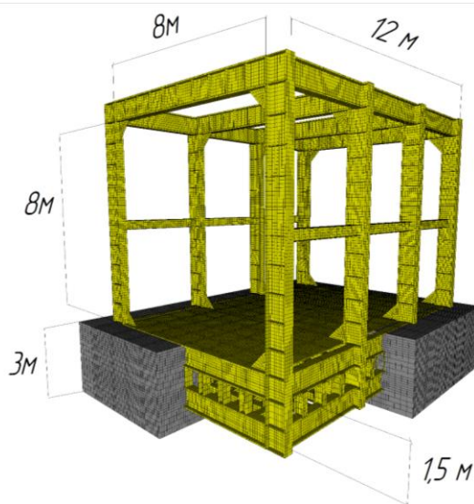
Рис. 3. Конструкция экспериментального стенда
