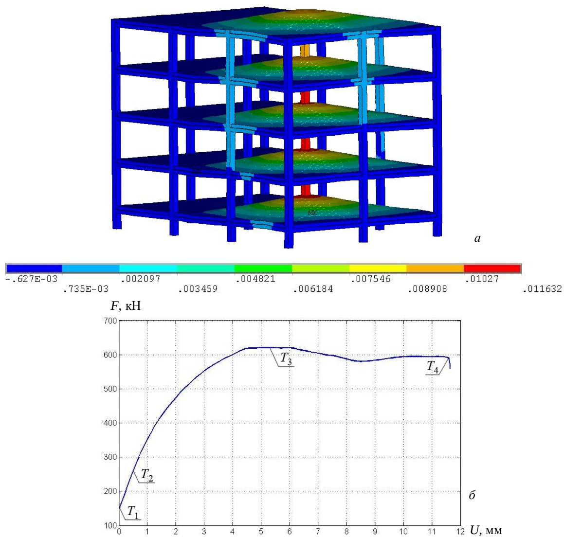
Рис. 2. Результаты моделирования: а – поле вертикальных перемещений; б – усилия, реализующихся в колонне в зависимости от приложенных перемещений (точками T_i обозначены ключевые состояния конструкции)
